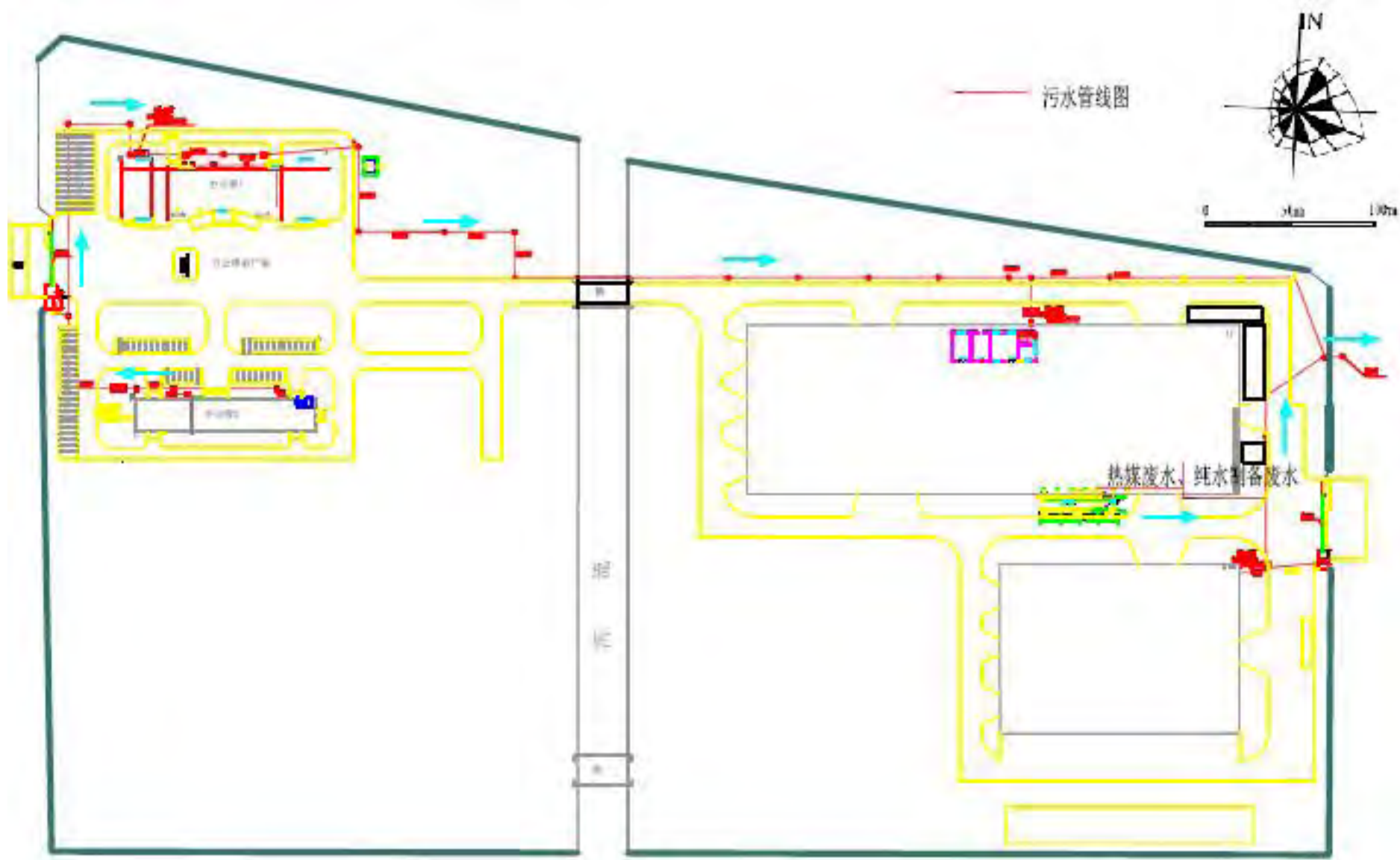
附图(7) 废水管网图
